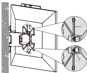
Fig. 43: Fissaggio dello schermo piatto
