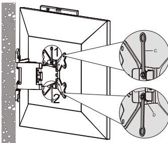
Fig.10: Anschrauben des Flachbildschirms
