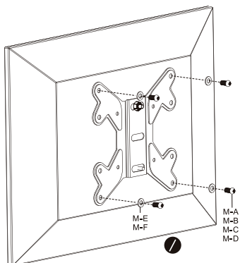
Fig. 40: Schermi piatti con fondo piatto
