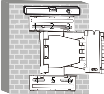
Fig. 2: Ausrichten und Anzeichnen
