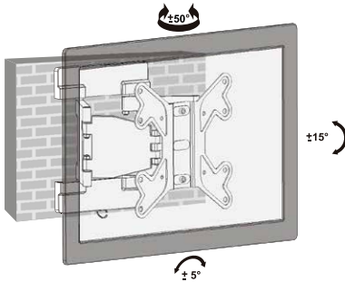
Fig. 11: Ausrichten des Flachbildschirms
