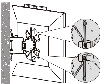
Fig.32: Vissez l'écran plat
