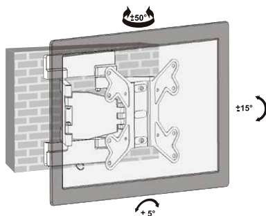
Fig.44: Allineamento dello schermo piatto
