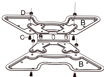
Fig. 39: Installazione dello schermo piatto
