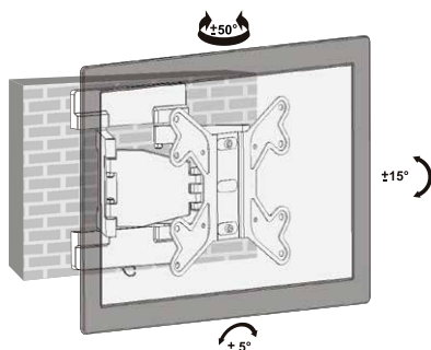
Fig.33: Ajuster l'écran plat
