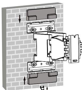
Fig. 38: Rimontare la coperchi in plastica
