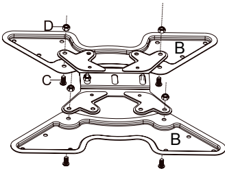
Fig. 6: Flachbildschirmmontage
