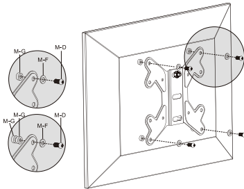
Fig. 8: Flachbildschirme mit gewölbter Rückseite
