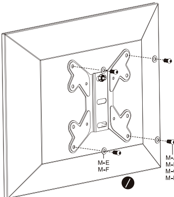
Fig. 7: Flachbildschirme mit flacher Rückseite
