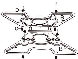
Fig.28: Montage de l'écran plat
