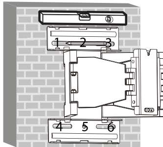
Fig.24: Alignement et marquage
