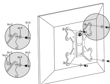
Fig. 30: Ecrans plats avec face arrière courbée
