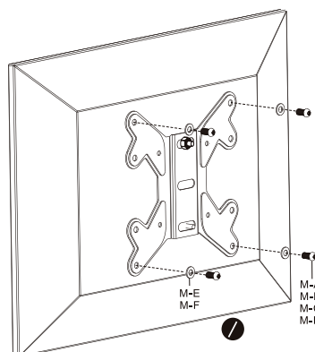
Fig. 29: Ecrans plats avec face arrière plane
